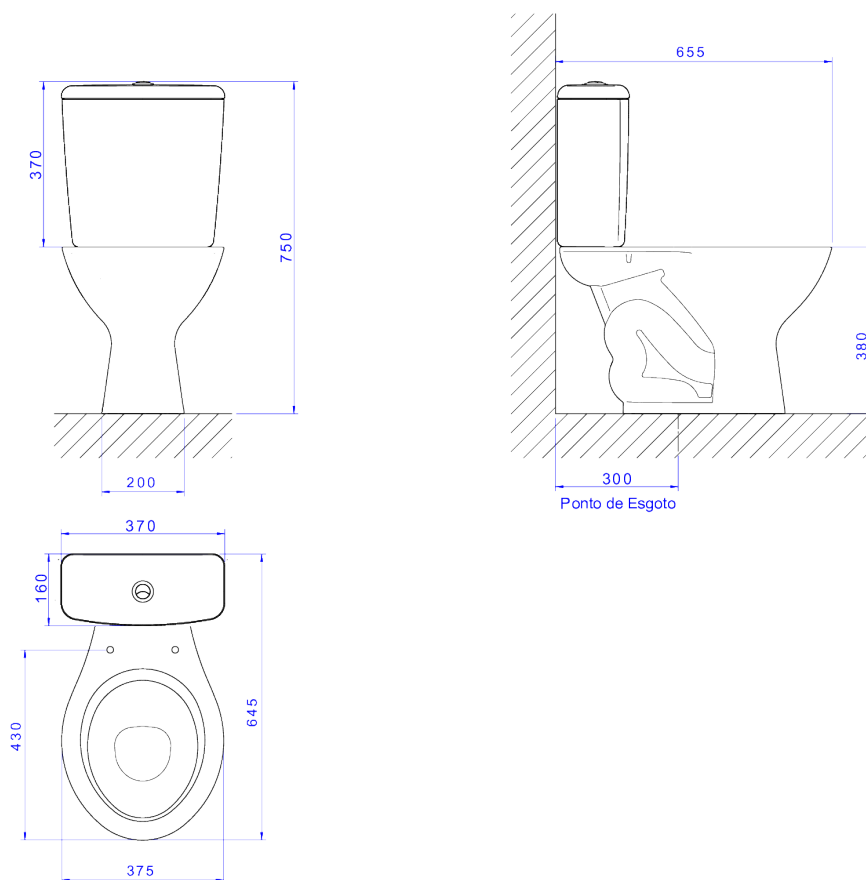
Desenho Técnico
